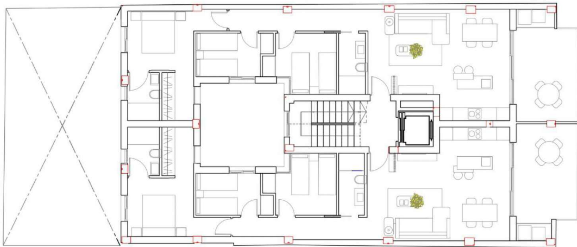
PLANTA 1-2-3
